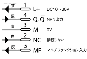
UM18-51115 M12-5ピン
