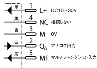
UM18-11116、-11117 M12-5ピン
