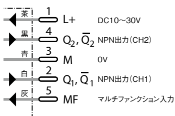
UM30-2□□□□4 M12-5ピン
