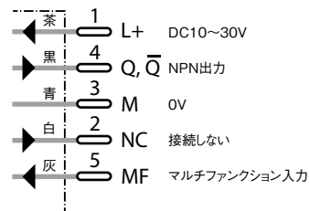
UM30-2□□□□5 M12-5ピン
